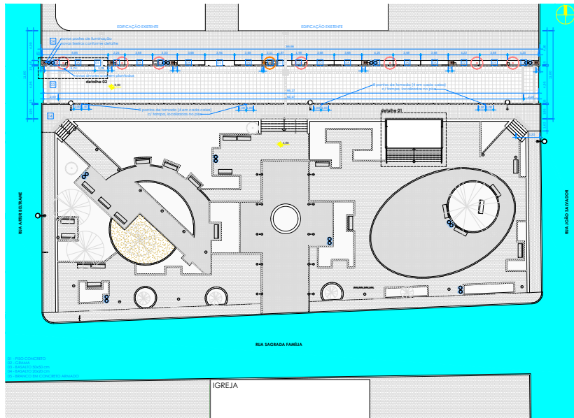
PAV. TÉRREO - PROJETO Escala: 1:200
