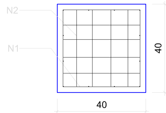
Bloco 12x PLANTA
