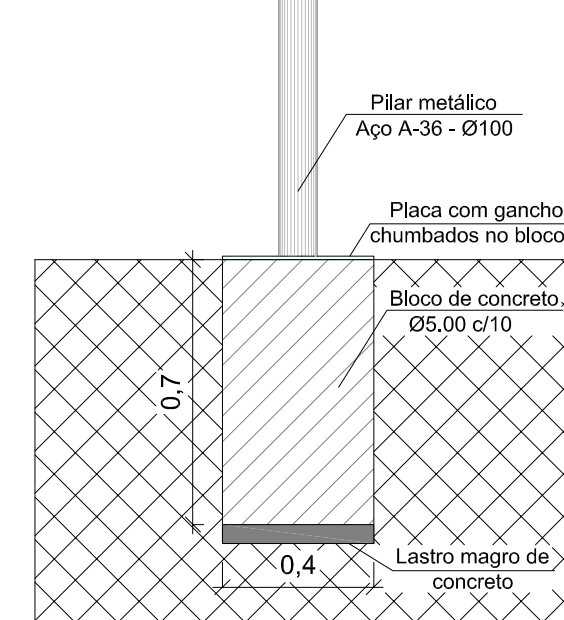
Detalhe Fundação Sem escala
