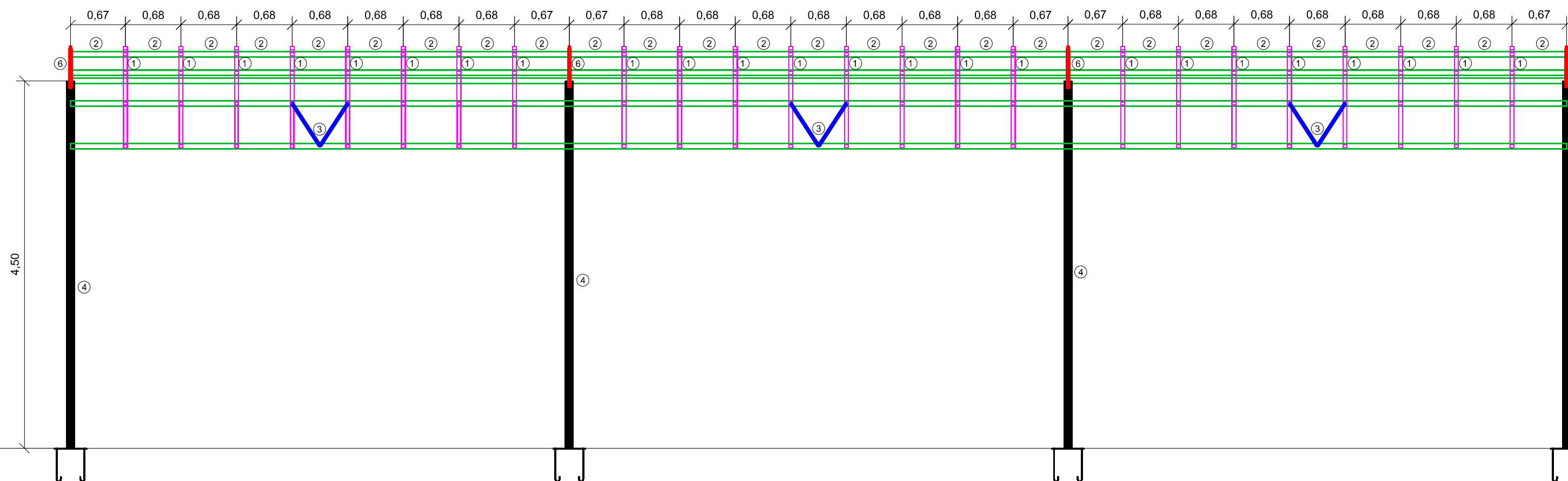
VISTA INTERMEDIÁRIA ESC: 1/50
