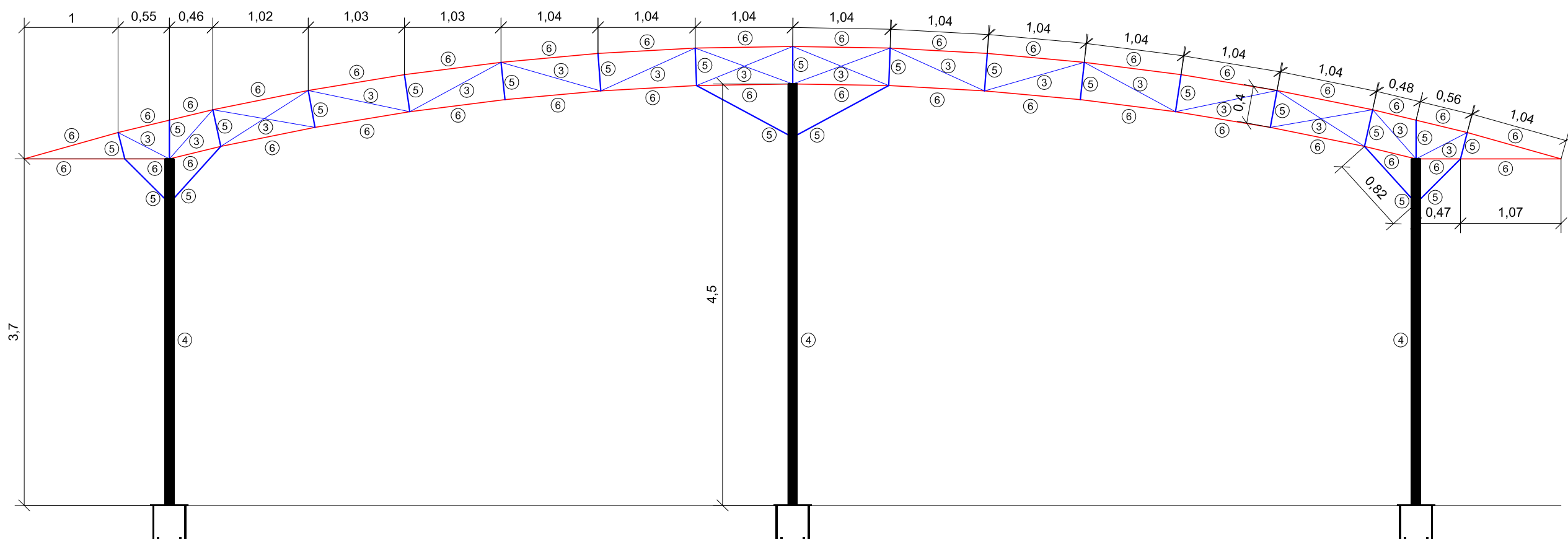
VISTA FRONTAL ESC: 1/50
