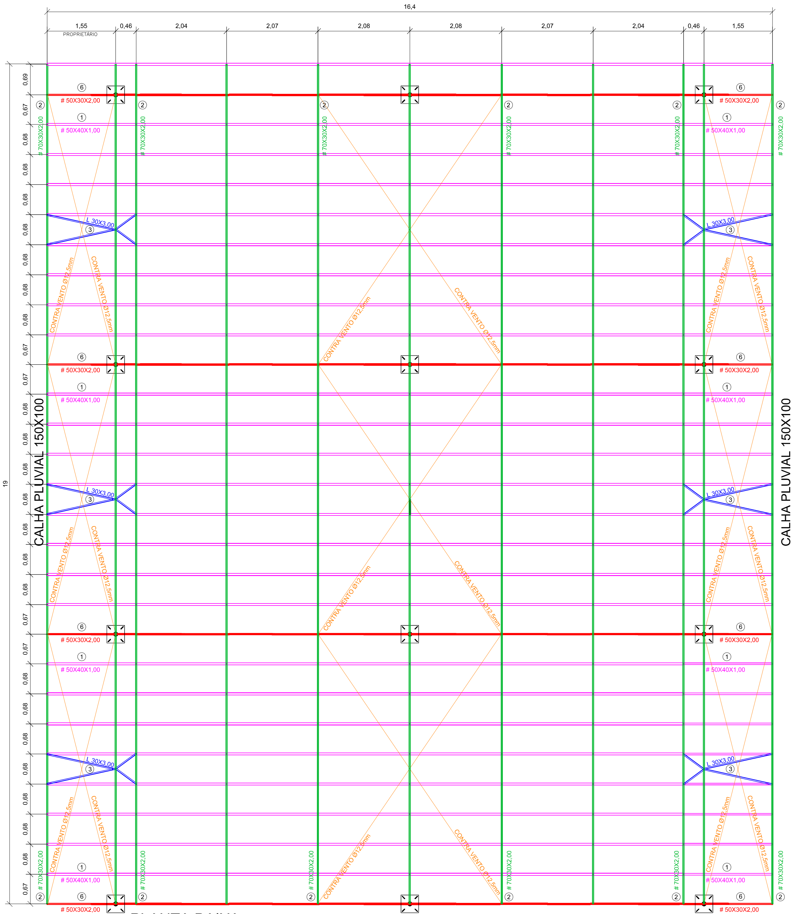
PLANTA BAIXA ESC: 1/50
